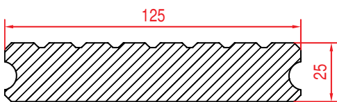
Thermo-Esche 25 x 125 mm, eins. gerillt, eins. glatt gehobelt, seitlich mit Seno-Profil
