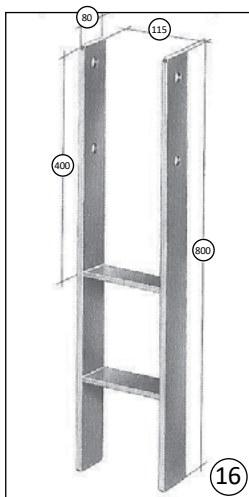
Metallschuhe H-Form, schwere Ausführung
