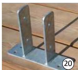
Metallschuhe zum Aufdübeln, besonders schwere Ausführung
