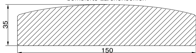
bombiert
