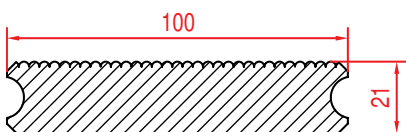
Thermo-Esche 21 x 100 mm, eins. fein geriffelt, eins. glatt gehobelt, seitlich mit Seno-Profil
